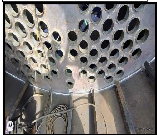
BAFLE SECCION-C-6
